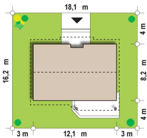
IŠDĖSTYMAS SKLYPE
